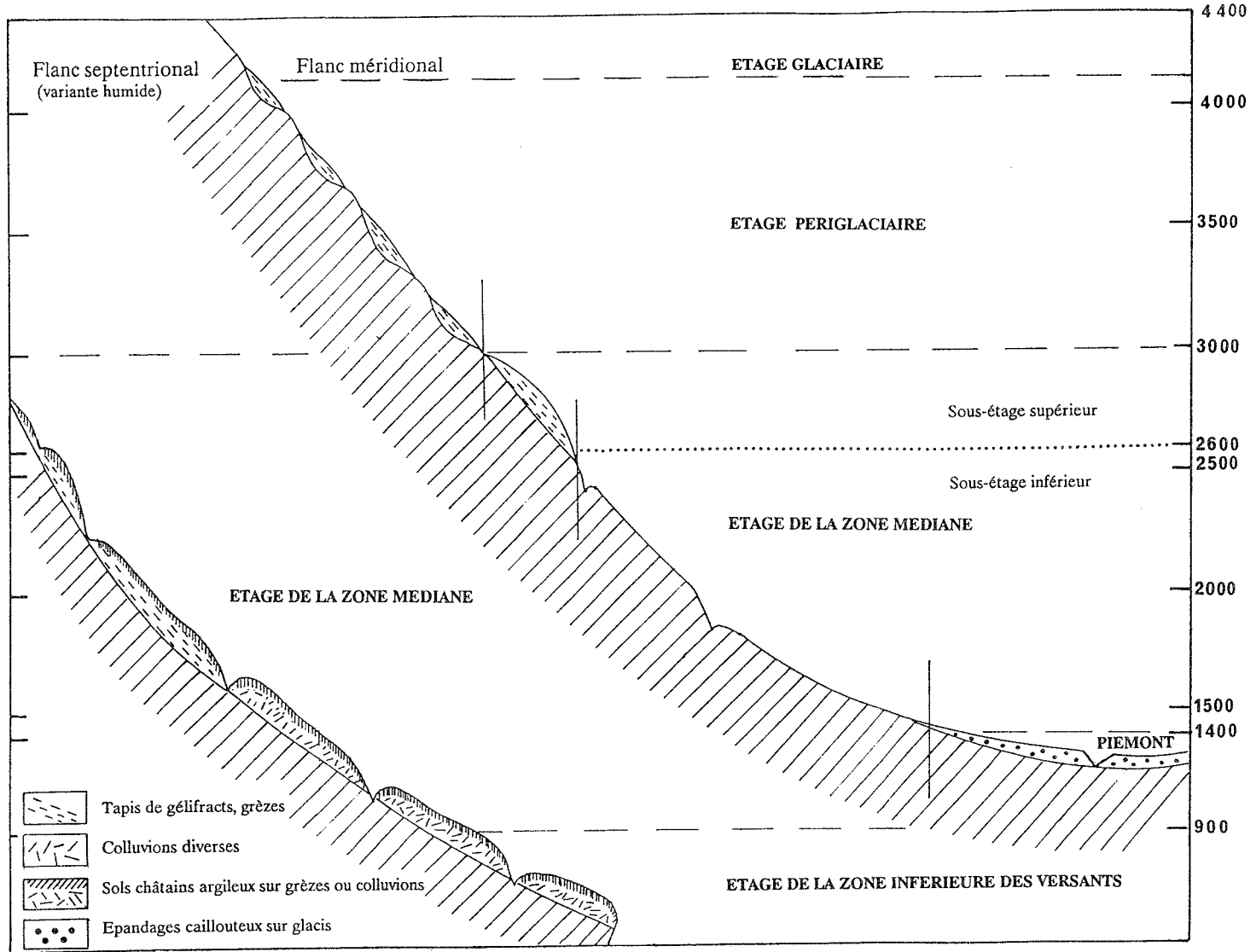
Fig. 6 : étages morphoclimatiques de l'Alborz (d'après RAYNAL, 1976)
