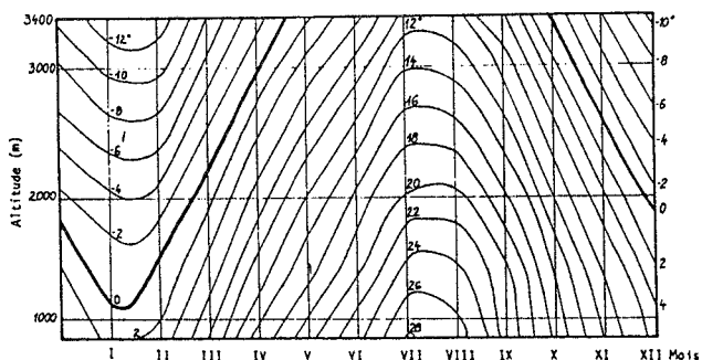
Fig. 37 : isothermes annuelles dans la vallée de Varzob ( idem , fig. 8, p. 26).
