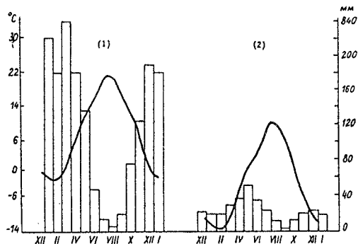
Fig. 35 : évolution annuelle des températures et des précipitations dans la vallée de Varzob (Khodza-Obi-Garm, 1807 m et Anzob, 3380 m) (OVCHINIKOV, 1971, fig. 7, p.p., p. 27).
