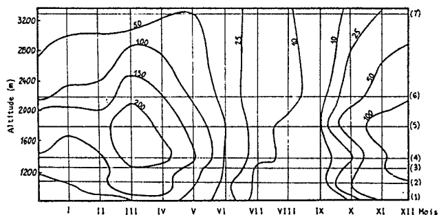
Fig. 36 : isohyètes annuelles dans la vallée de Varzob (stations de Doshanbé (1) ; Varzob (2) ; Pugus (3) ; Gushary (4) ; Khodza-Obi-Garm (5) ; Ziddy (6) ; Anzob ( idem , fig. 9, p. 27)).
