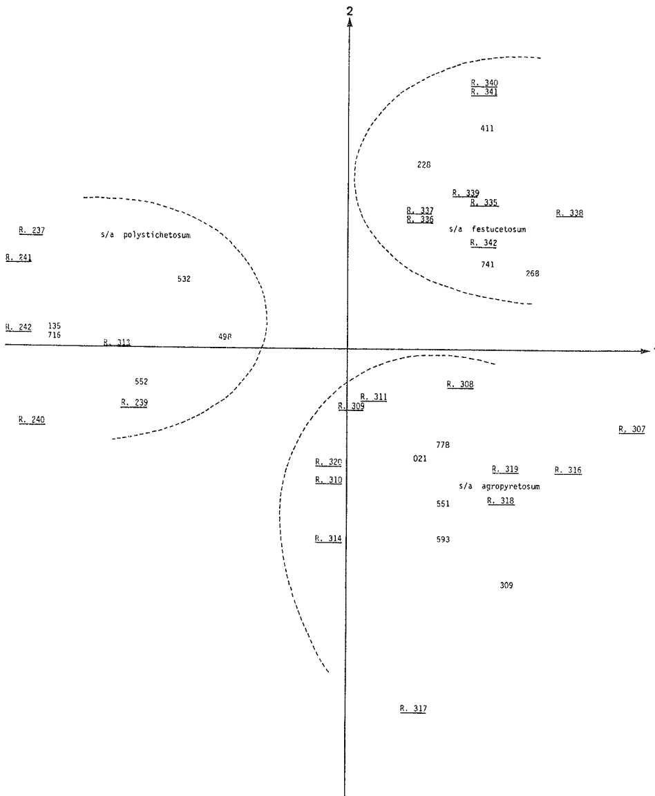
Fig. 32 : analyse partielle de l'ACERI HYRCANI-QUERCETUM MACRANTHERAE. Carte des relevés et des espèces selon les axes 1-2 (avec figuration des seules différentielles).
