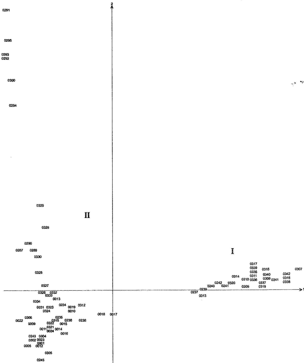
Fig. 30 : analyse globale des groupements subalpins forestiers (I) et des pelouses voisines (II). Carte des relevés selon les axes 1-2.
