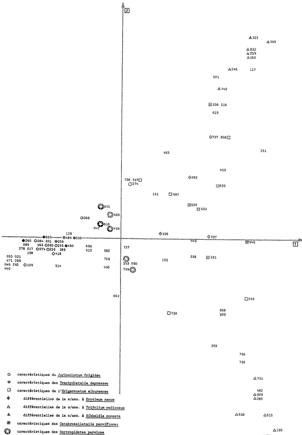
Fig. 28 : analyse des pelouses alpines supérieures du JURINETUM FRIGIDAE et de l' ERIGERONETUM ELBURSENSIS . Carte des espèces selon les axes 1-2.
