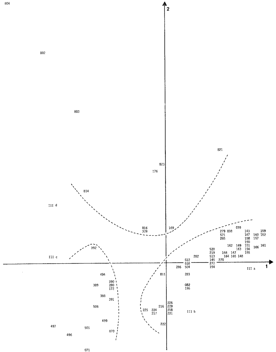
Fig. 24 : analyse partielle portant sur l'ensemble III (pelouses alpines inférieures de l' IRIDETUM BARNUMAE ). Carte des relevés selon les axes 1-2.
